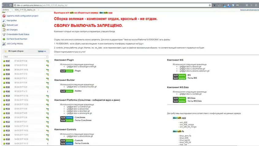
Рисунок 3. SDK.
